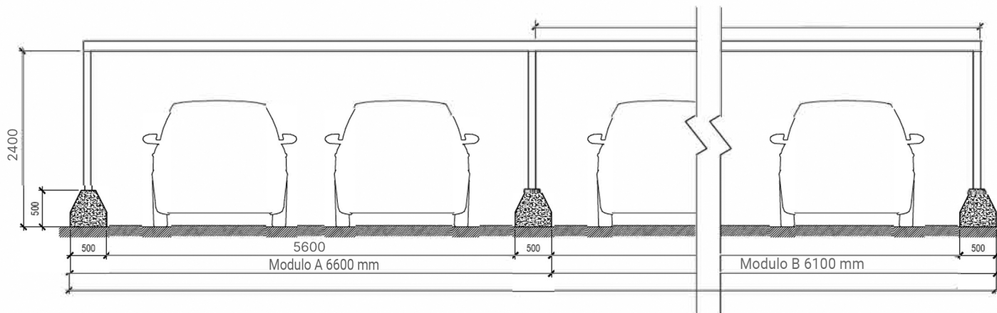
VISTA FRONTALE
