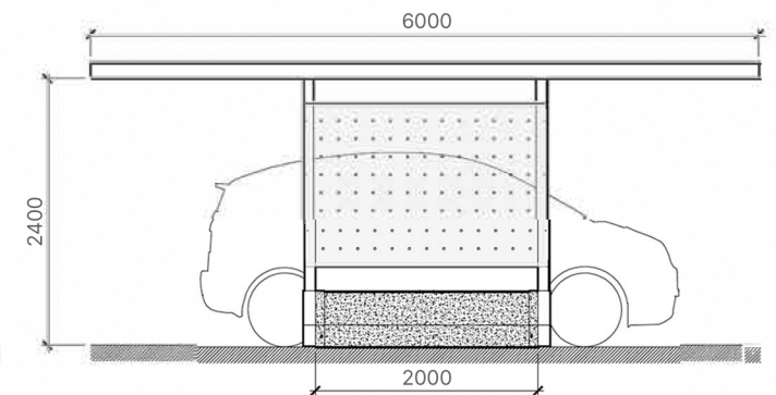
VISTA LATERALE
